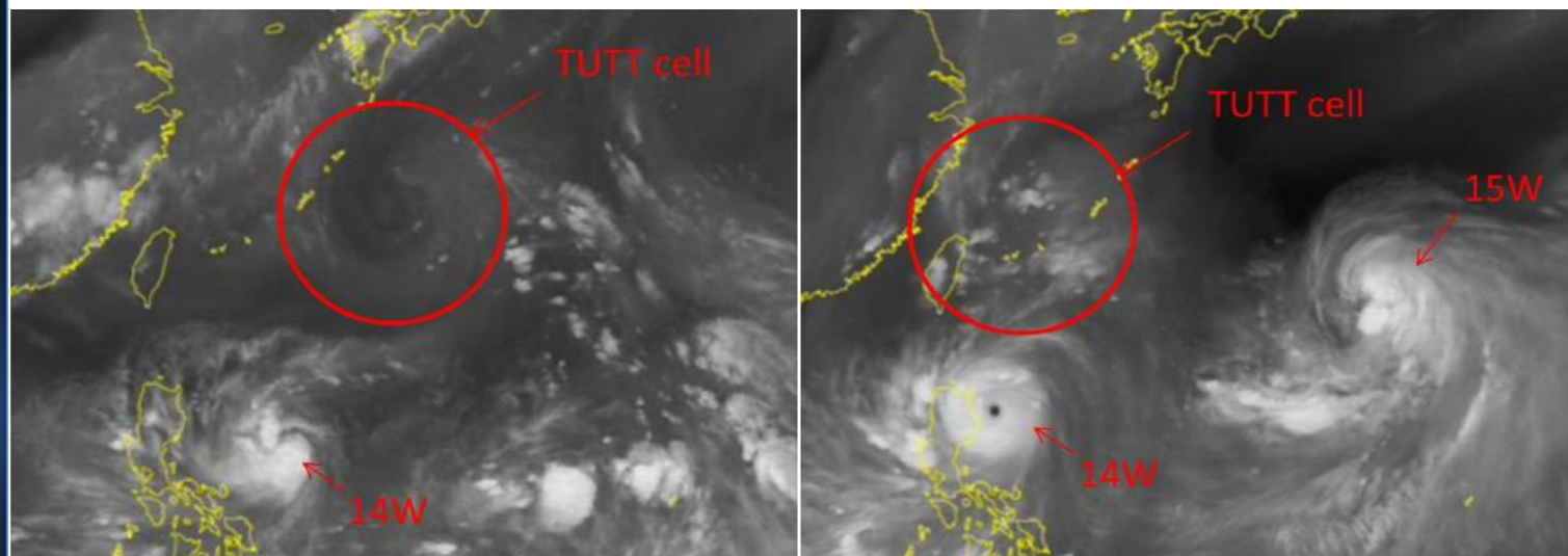
2011年8月23日20时水汽云图
